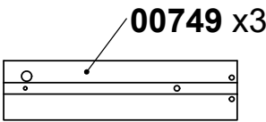
345x88x12,2mm
